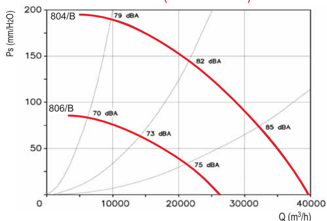
ROOF-HP 800/B (F400 - F600)
