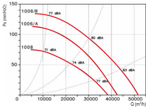
ROOF-HP 1000 (F400 - F600)
