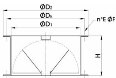
(GS-RH) Serranda gravità/Gravity shutter
