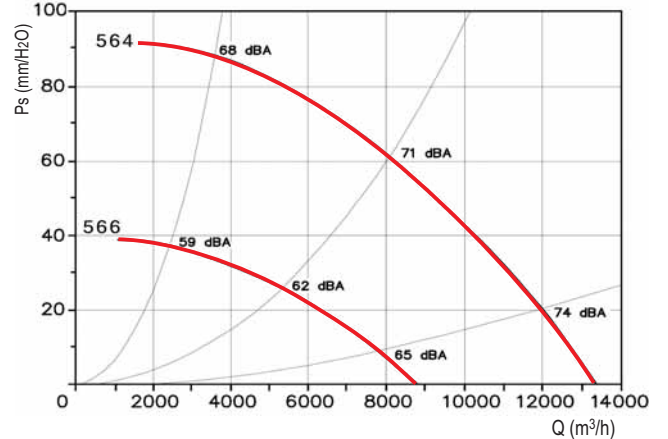
ROOF-HP 560 (F400 - F600)
