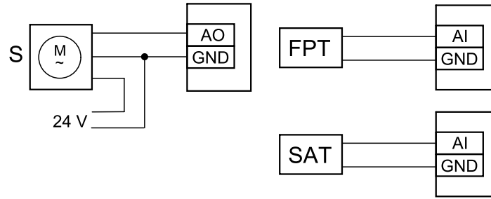
Kuva 15 Lämminvesipatterin kytkennät
