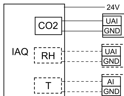
Bild 13 Anbindung IAQ Sensoren
