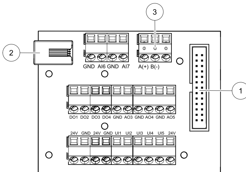
Bild 6 Außenliegenden Anschlussbox und Platine.
