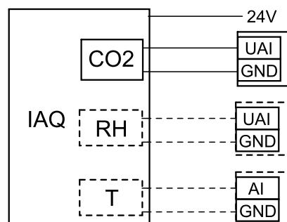
Kuva 13 IAQ liitännät
