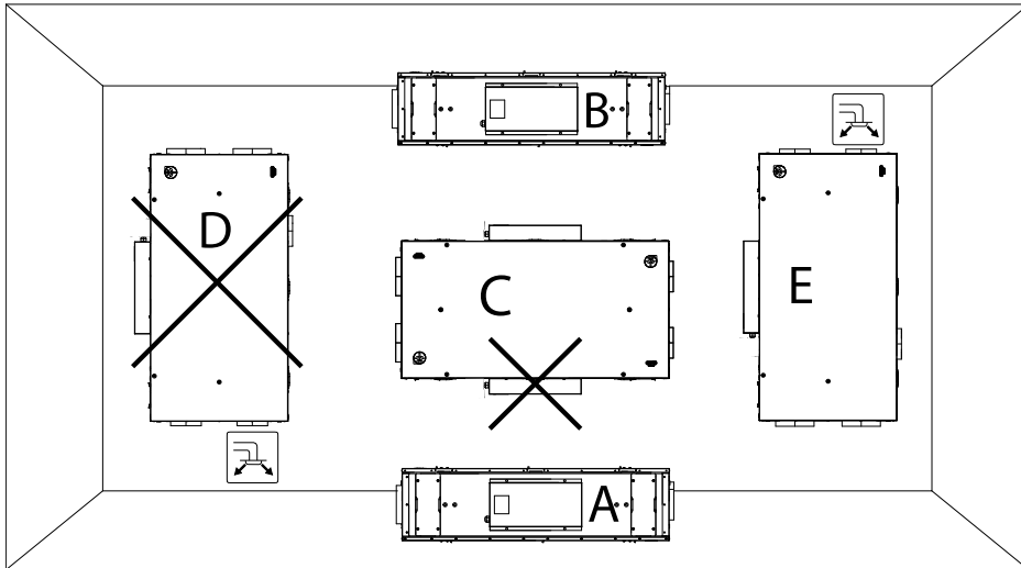
Fig. 3 Möjliga installationspositioner
