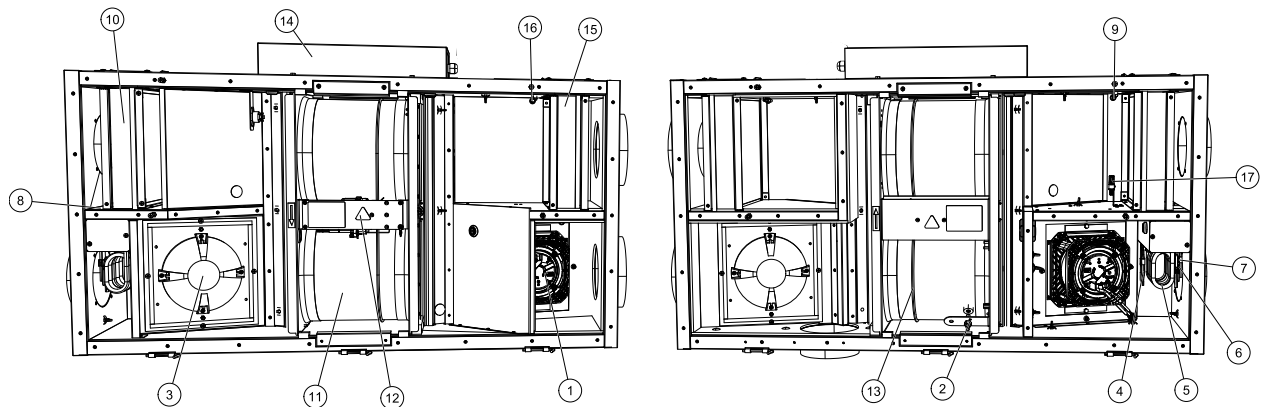
Kuva 10 Sisäiset komponentit
