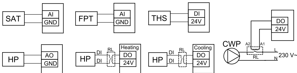
Fig. 17 Växlande uppvärmnings-/kylningsanslutningar
