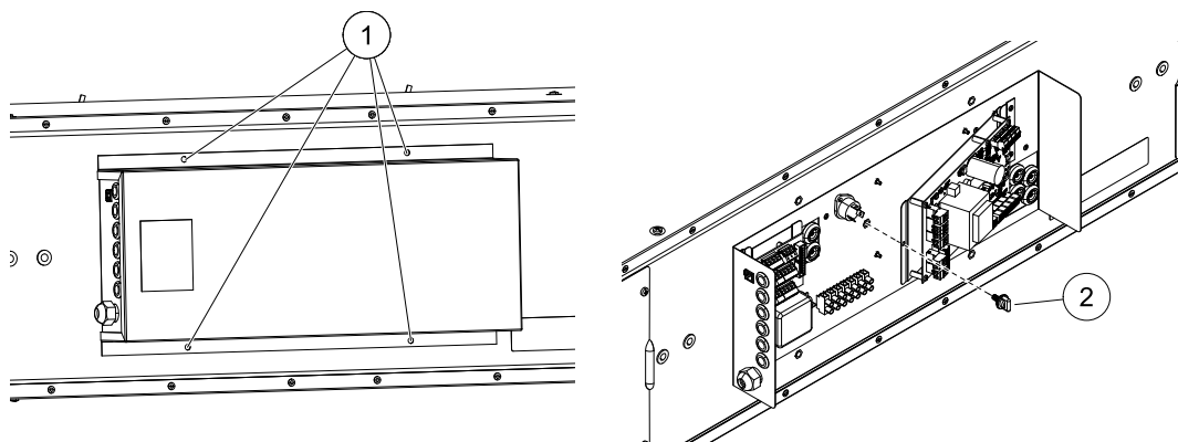
Fig. 4 Kretskort
