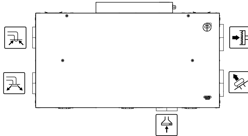
Bild 2 Kanalanschlüsse
