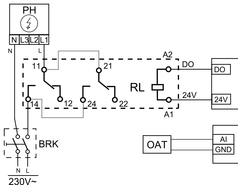
Bild 14 Anbindung Vorheizregister
