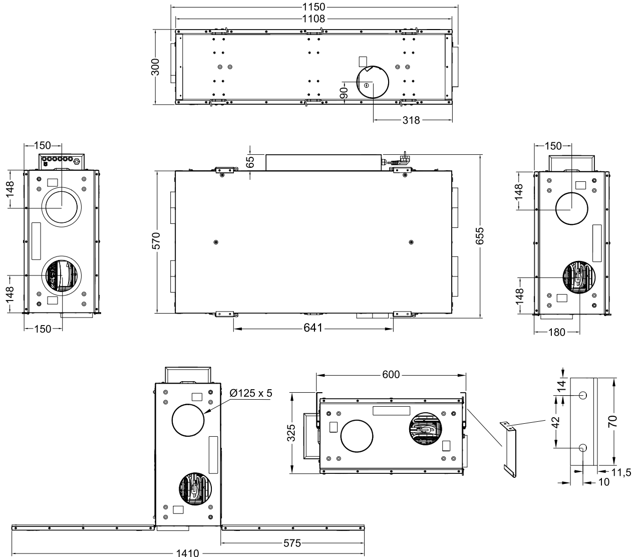
Fig. 1 Mått
