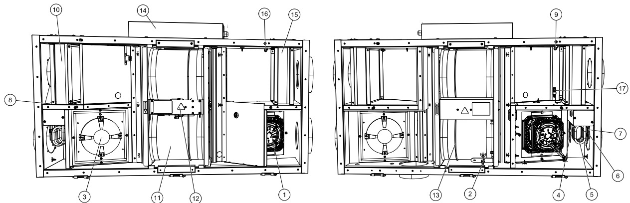
Bild 10 Interne Komponenten
