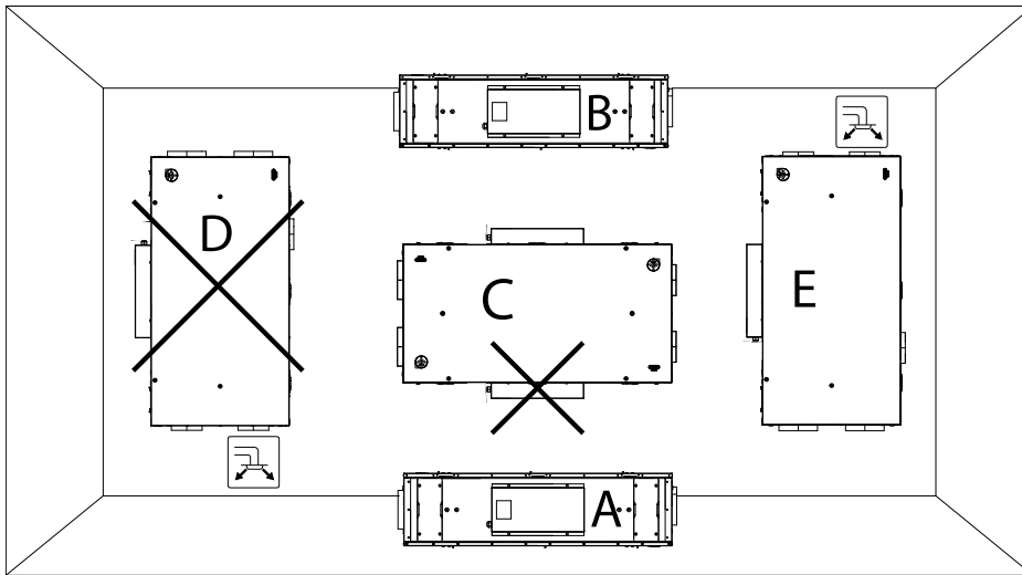
Kuva 3 Mahdolliset asennusasennot
