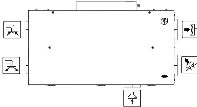
Kuva 2 Kanavaliitännät
