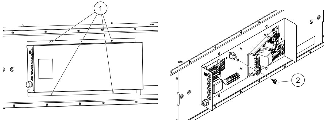
Kuva 4 Piirikortti
