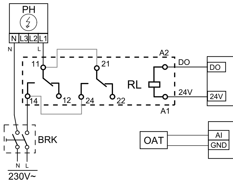
Kuva 14 Etulämmittimen konfigurointi
