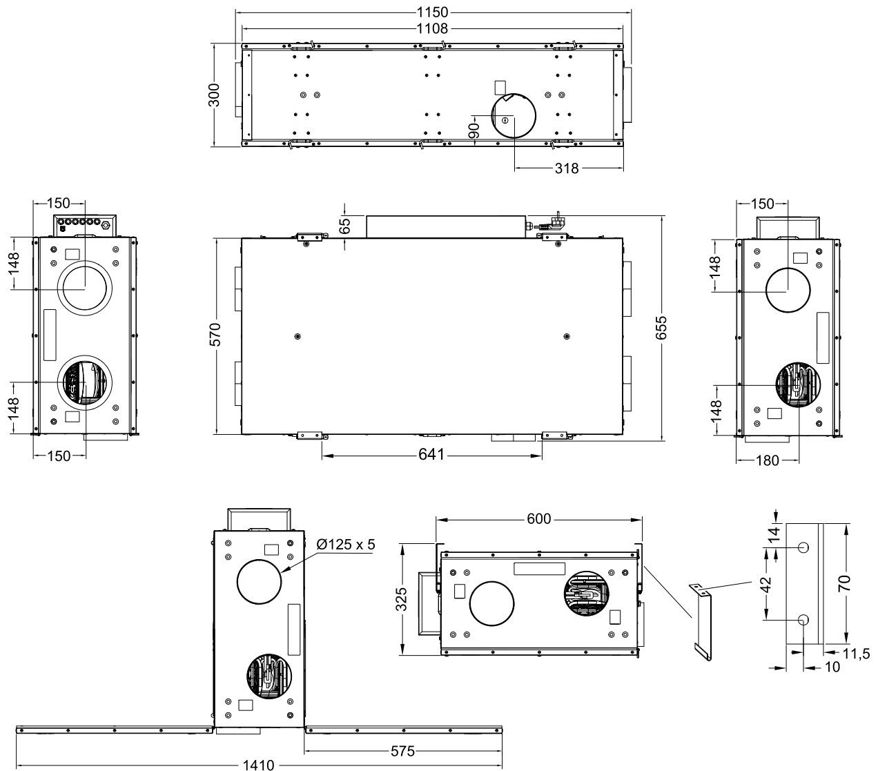
Bild 1 Abmessungen
