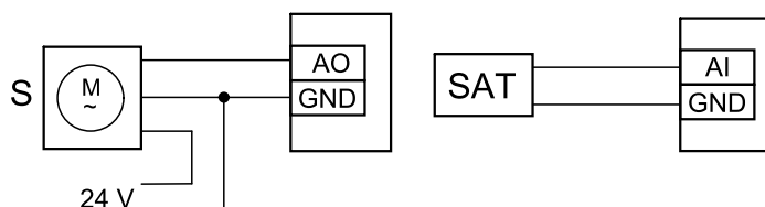
Bild 16 Anbindung Kanalkühlregister
