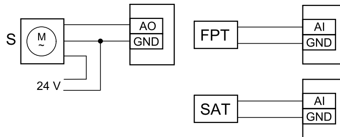
Bild 15 Anbindung Wassernachheizregister
