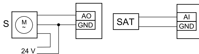
Fig. 16 Kanalkylaranslutningar
