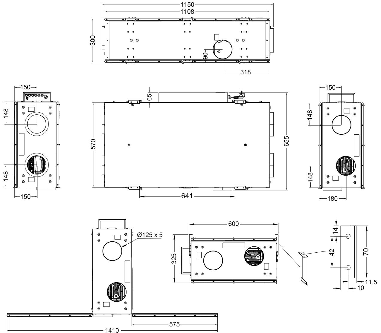
Fig. 1 Dimensions
