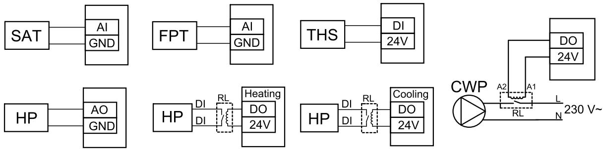
Kuva 17 Yhdistelmäpatterin liitännät
