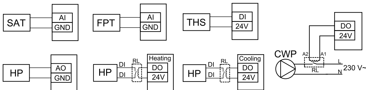
Bild 17 Anbindung DX-Heiz-/Kühlregister
