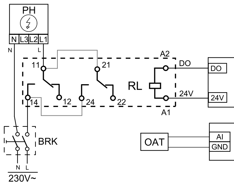
Fig. 14 Förvärmaranslutningar
