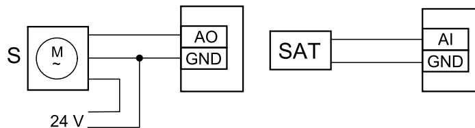
Kuva 16 Kanavajäähdyttimen liitännät
